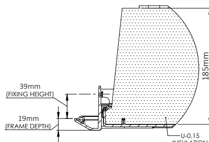
LT0015 | LT0015KL
