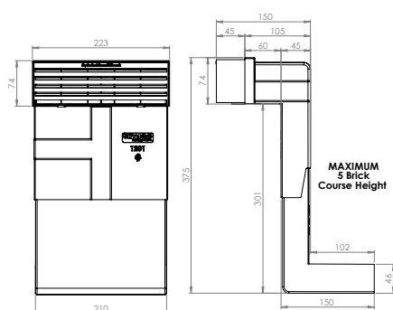
1201 DIMENSIONS
